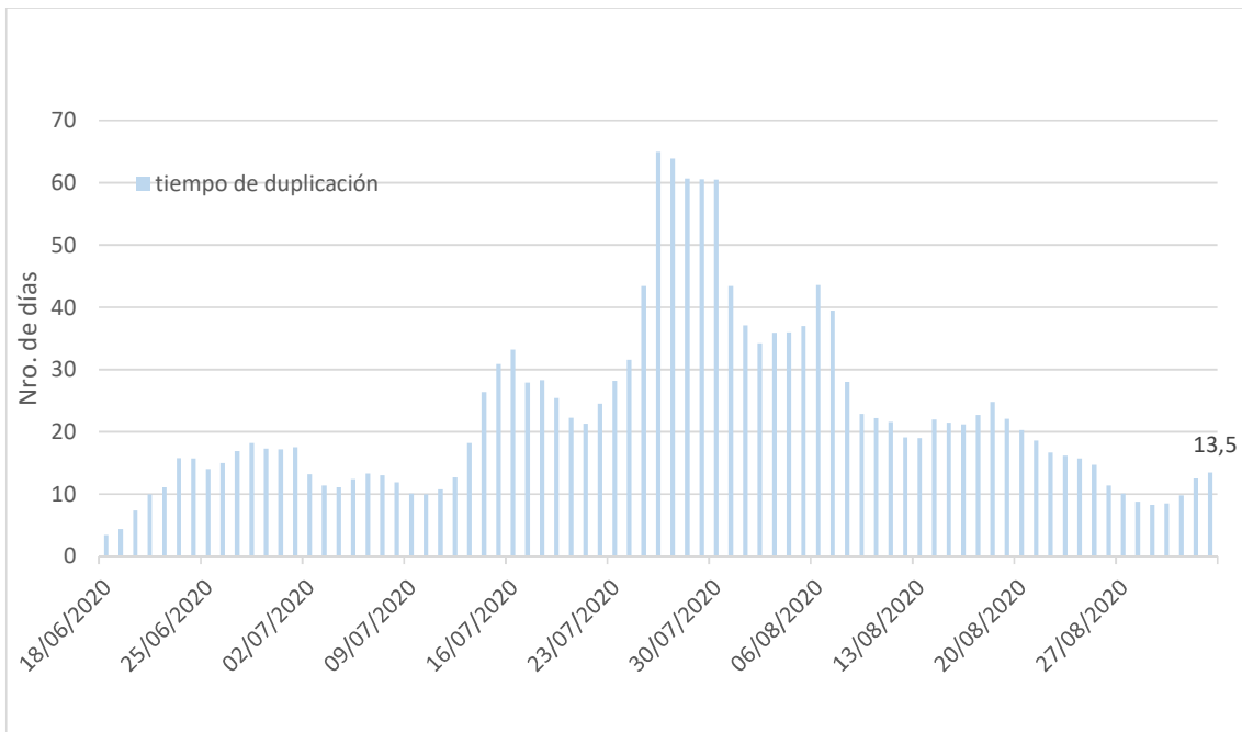
Tiempo de duplicación de Casos de Covid19 en AP Comodoro Rivadavia. Junio -Agosto 2020
